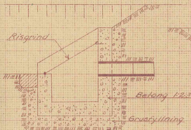
g Inloppsskydd med slambassäng
