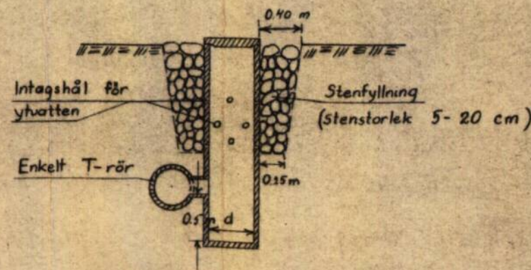
Brunn typ Aa vid sidan av rörledning
