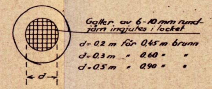
Detaljritning för lock med hål
