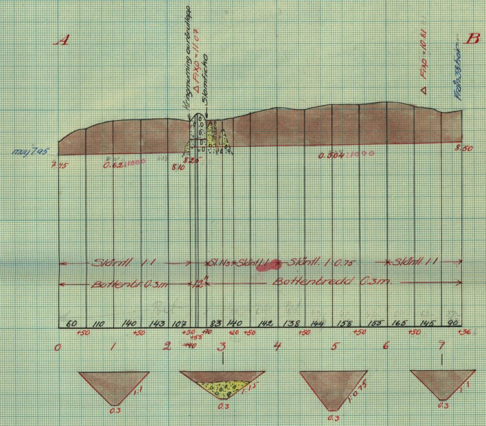
Kringmurning av rörutlopp vid 2+40
