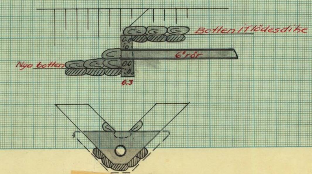
Kringmurning av rörutlopp vid 21
