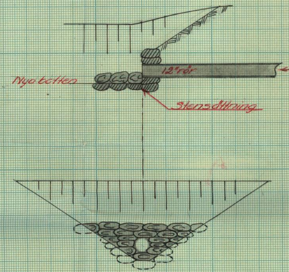
Kringmurning av rörutlopp vid 2+40
