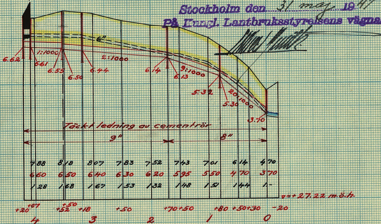
Förslag till ommurning av rörutlopp vid 0.
