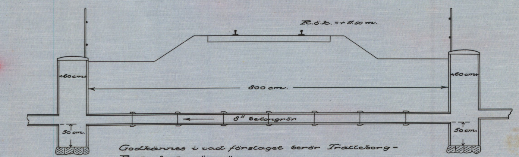
Förslag till rörledning genom järnväg.
