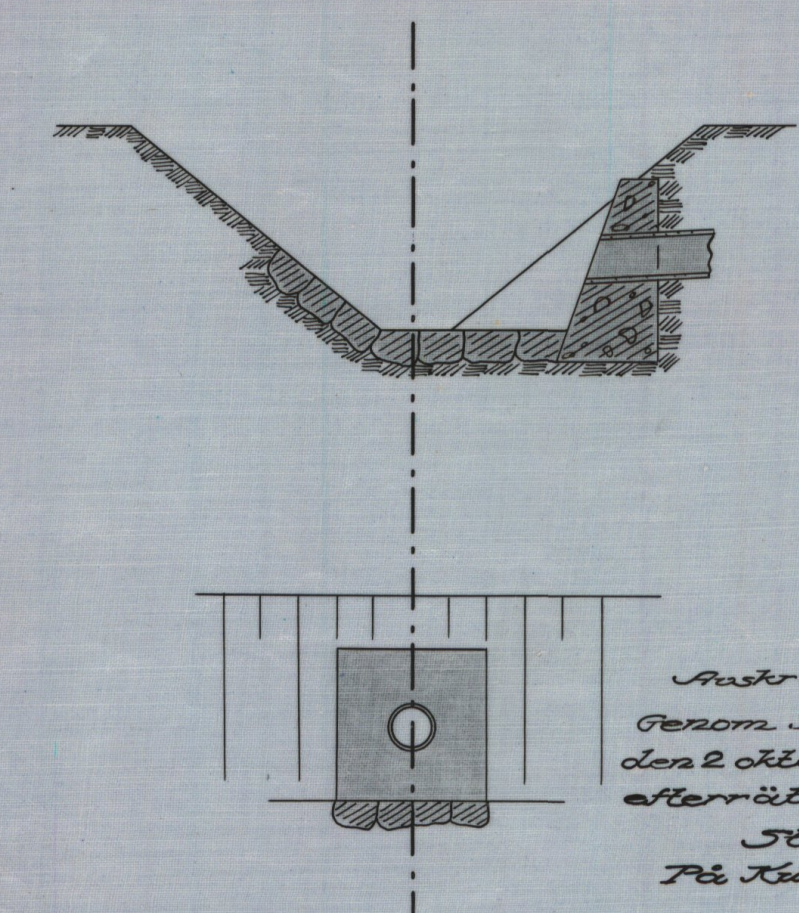
Förslag till rörutlopp vid A.
