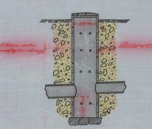
Typritning för brunnen
