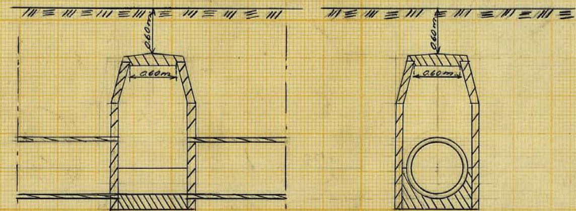
Förslag till 36" kopplingsbrunn.
