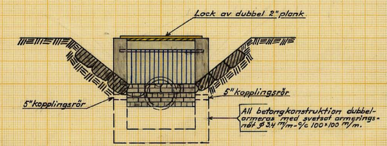
Typritning för intag vid 37+28. Skala 1:50.
