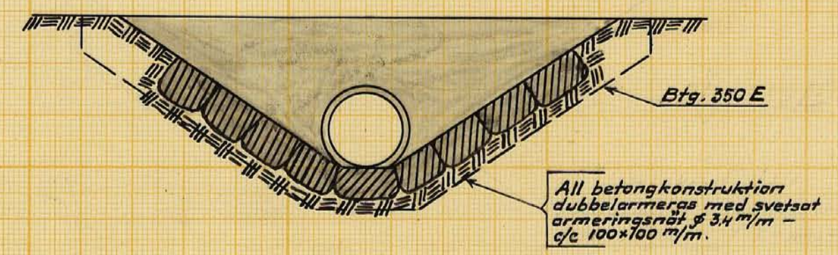
Typritning för ommurning vid 10+50. Skala 1:50.
