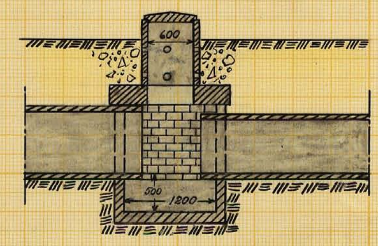
Typritning för brunn med 48" inre diameter. Skala 1:50.
