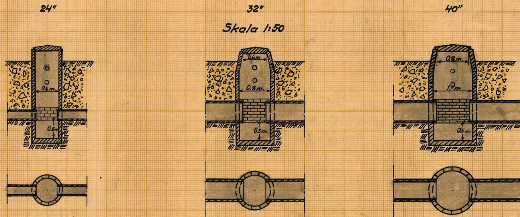
Typritningar för brunnar med inre diameter av:
