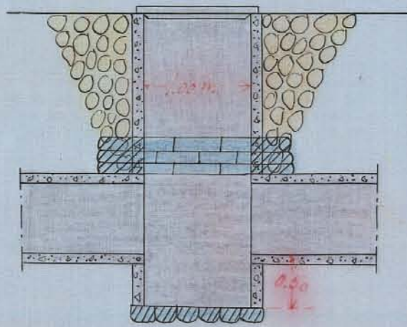
Förslag till intagningsbassäng
