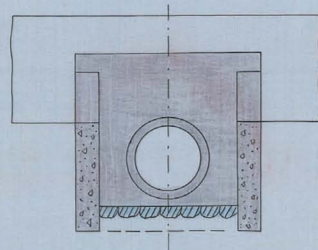
Förslag till dikesöga vid punkt 0.
