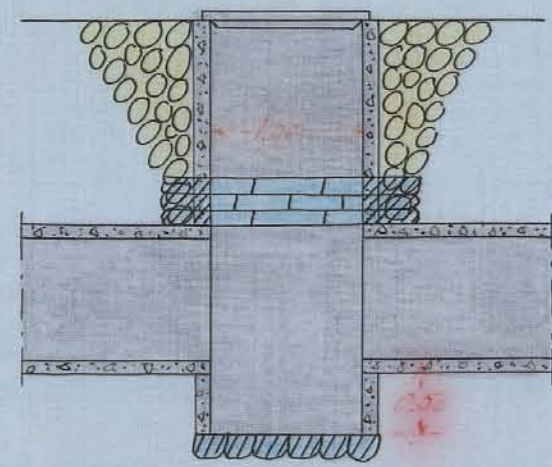
Förslag till intagningsbassäng vid punkt 16+30.
