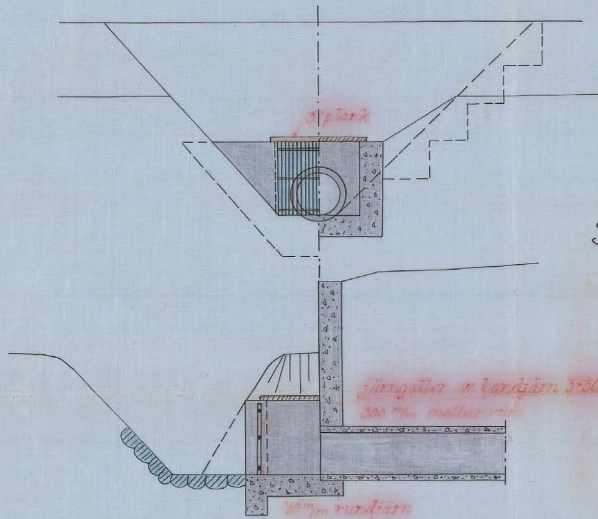
Förslag till intagningsbassäng vid punkt 16+30.
