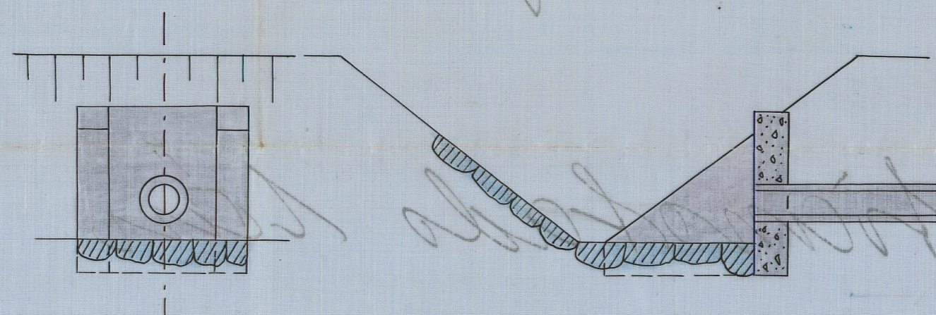
Förslag till dikesöga.
