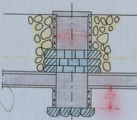
Förslag till intagningsbrunn.
