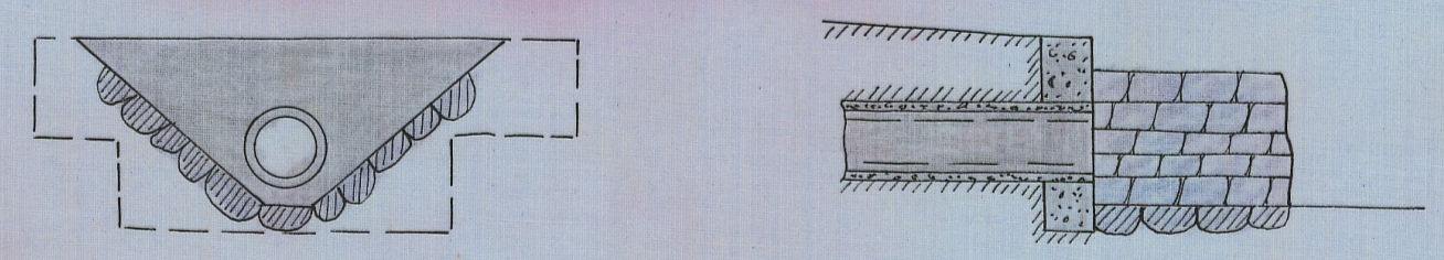
Alt II Förslag till dikesöga vid 3+58
