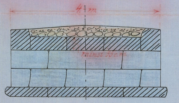
Alt I Förslag till ågavägsströmna vid 2+50
