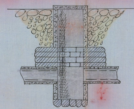
Alt II Förslag till intagningsbrunn
