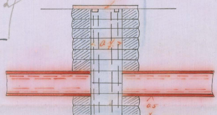
Förslag till dränsöga
