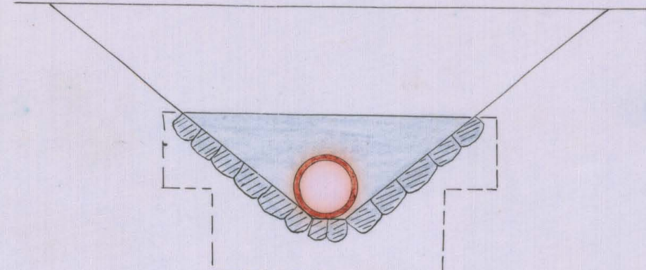
Förslag till dränsöga
