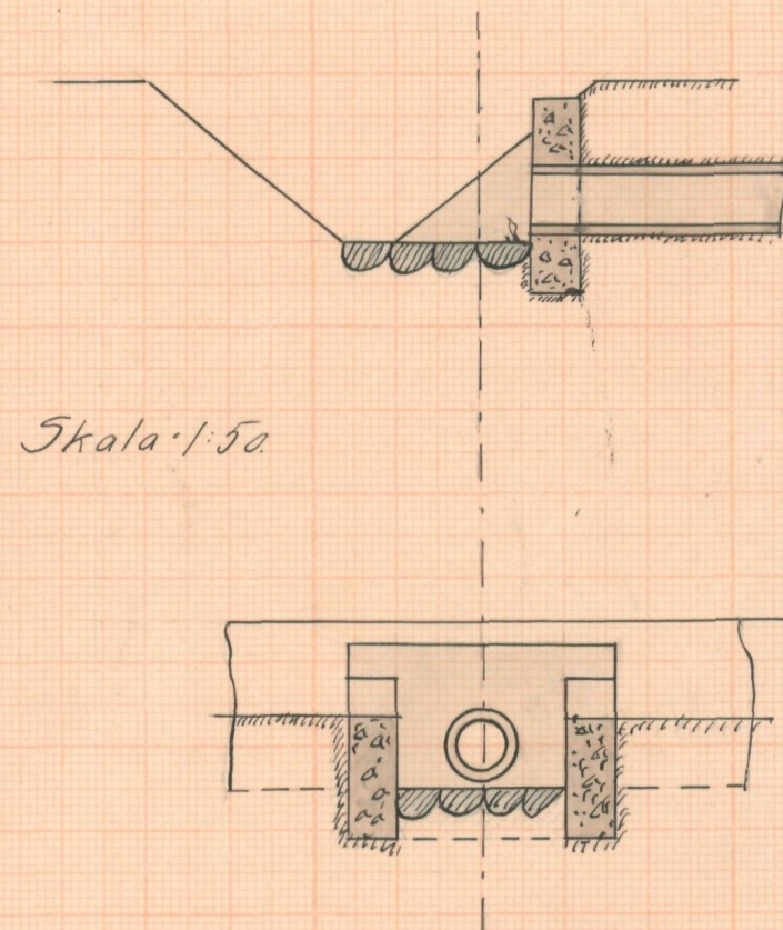
Förslag till dikesöga vid punkt O.
