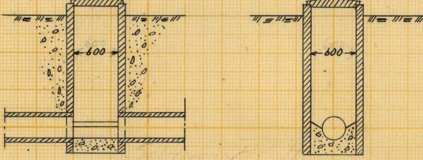
Typritning för 24" brunnar 1:50
