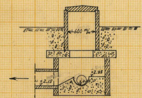
Sektion B-B
