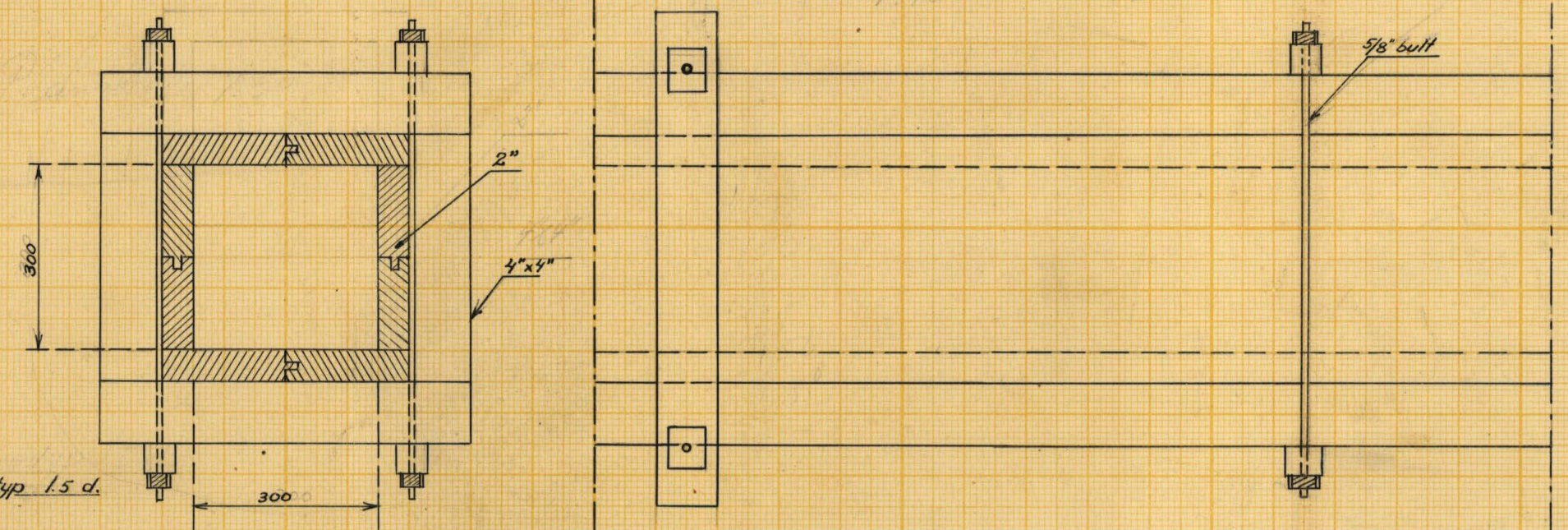
Detalj av utloppsledning Skala 1:10
