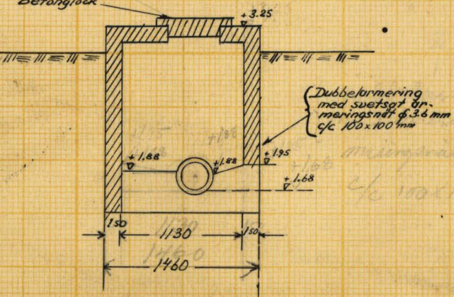
Sektion D-D
