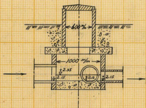
Sektion A-A
