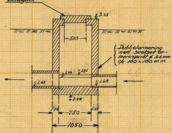
Sektion D-D
