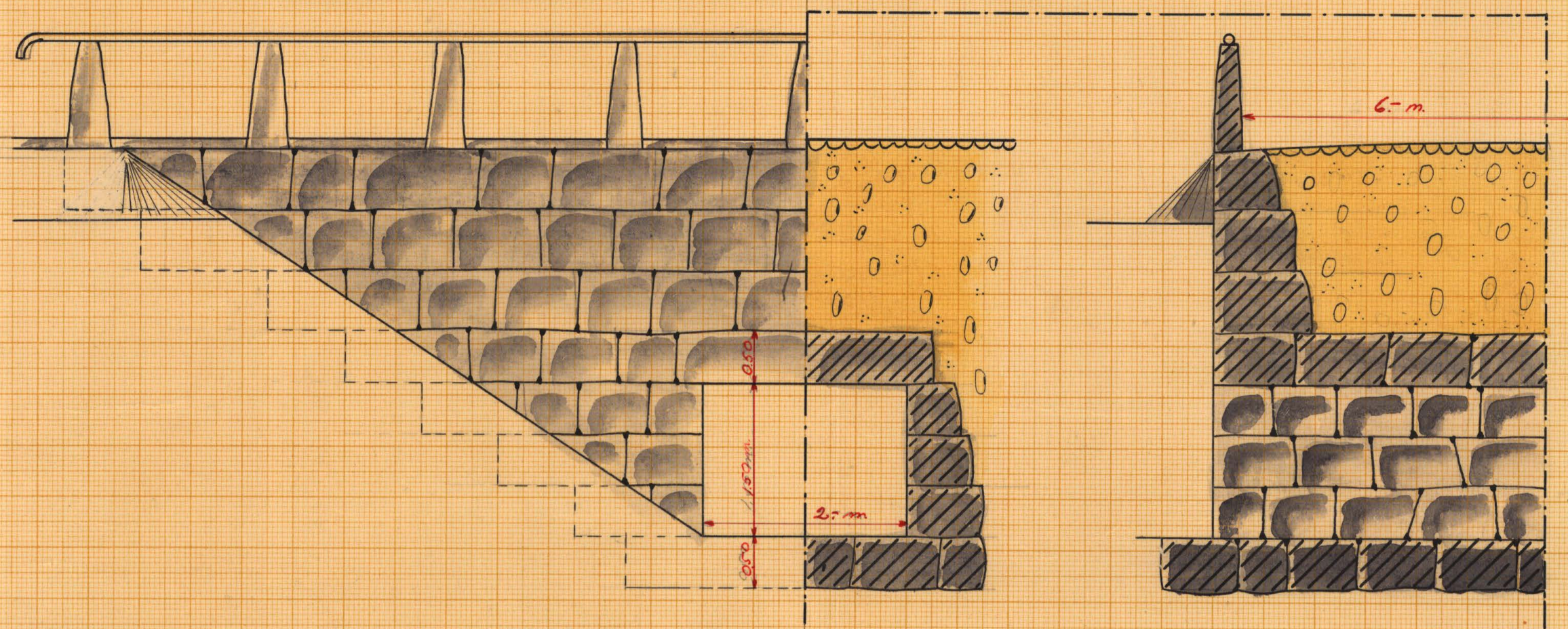
Förslag till ombyggnad av landsvägsbron vid 17+60.
