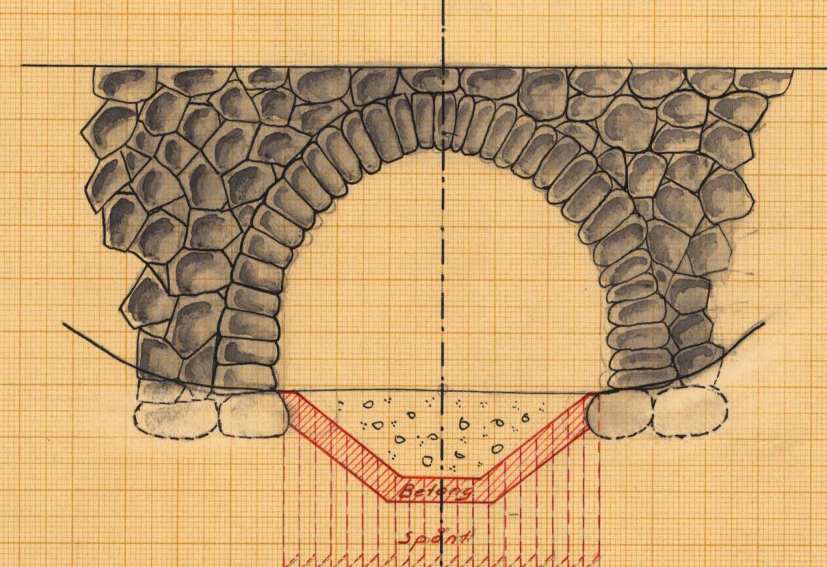
Förslag till underbyggnad av landsvägsbron vid 17+60.
