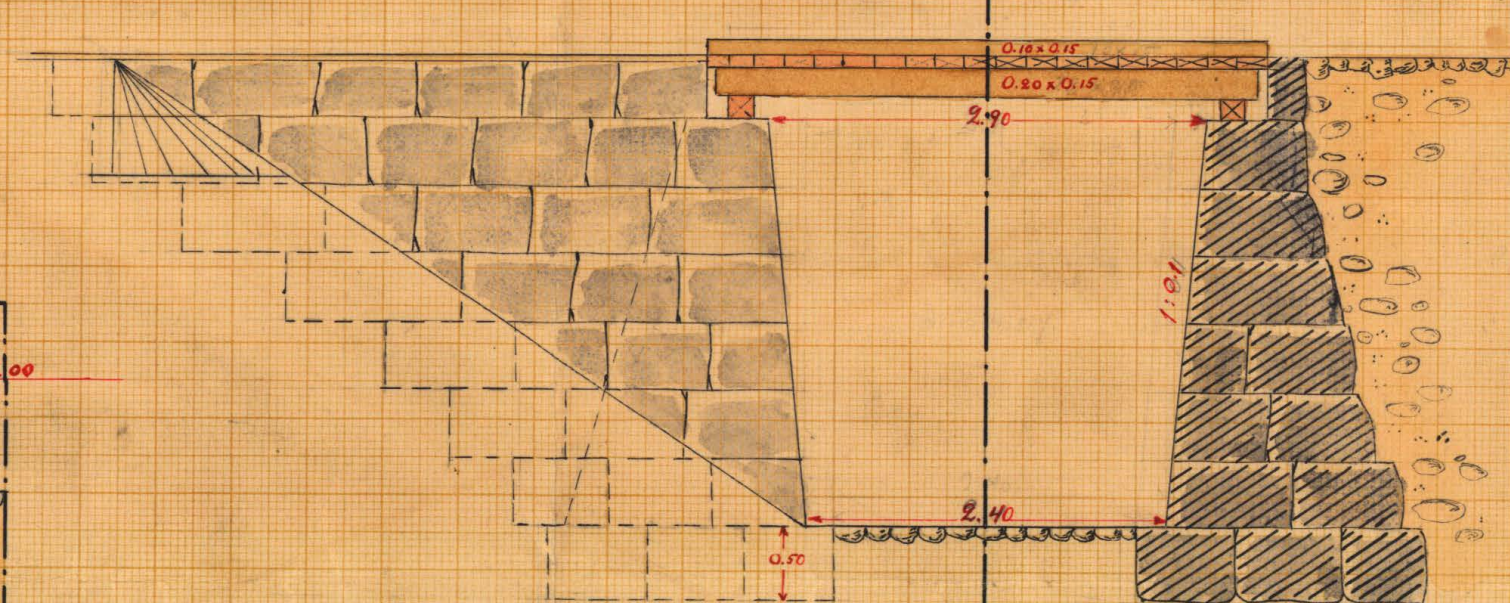
Ågövägsbro vid 12+72 (och 14+20).
