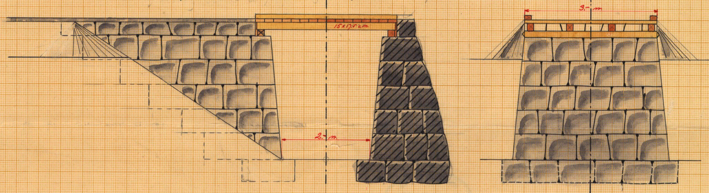
Alternativt förslag till utfartsvägsbroar vid 12+72 och 14+20.
