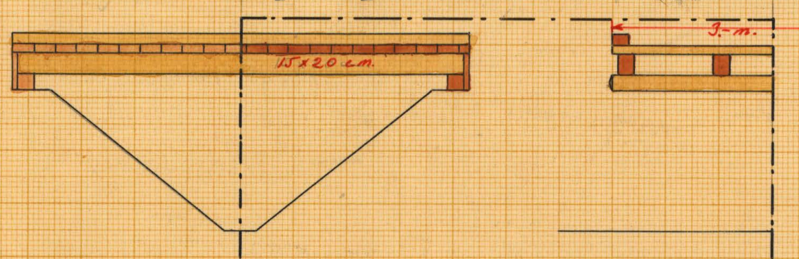
Förslag till ägrovägsbroar å sträckan C-E.
