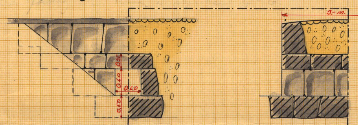
Alternativt förslag till trumma å sträckan C-E.
