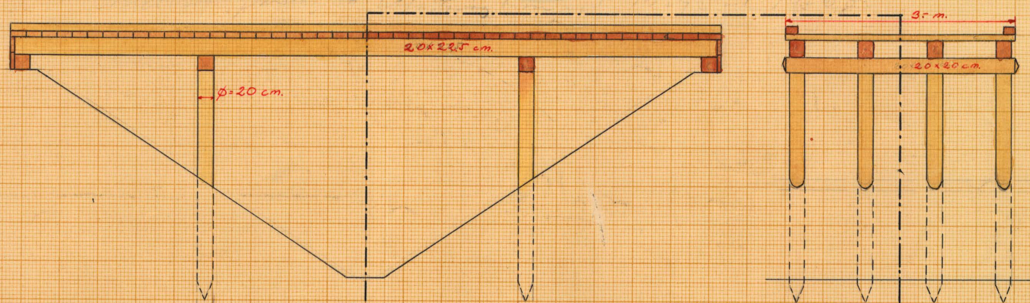
Alternativt förslag till utfartsvägsbroar vid 12+72 och 14+20.
