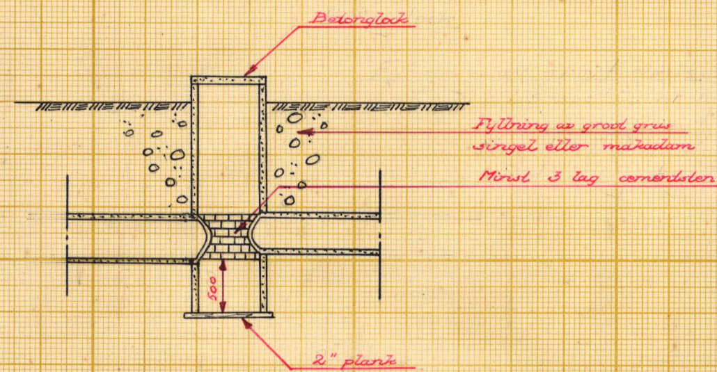
Förslag till kringmurning av rörulopp vid 12"00
