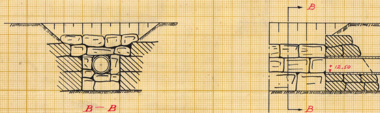
Förslag till kringmurning av rörulopp vid 12"00
