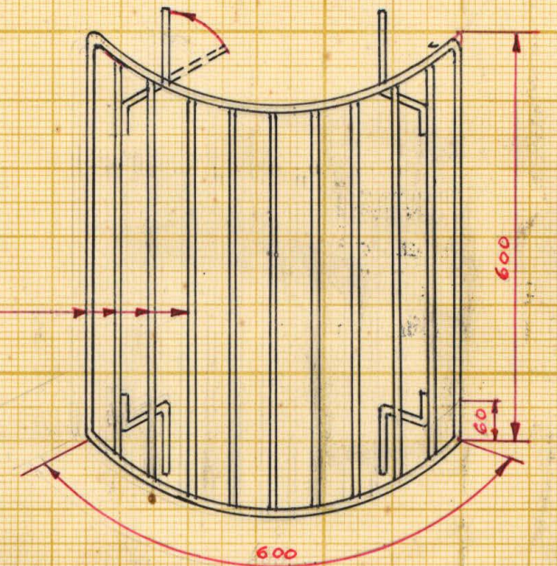
Delutg av galler Skala 1:10
