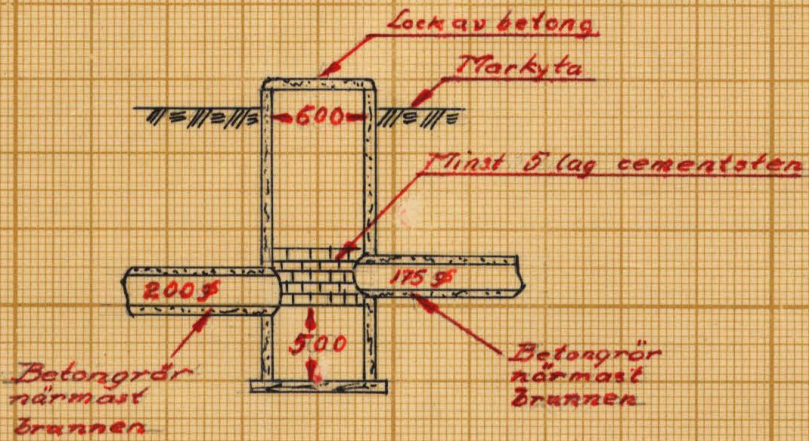
Typritning för brunnar
