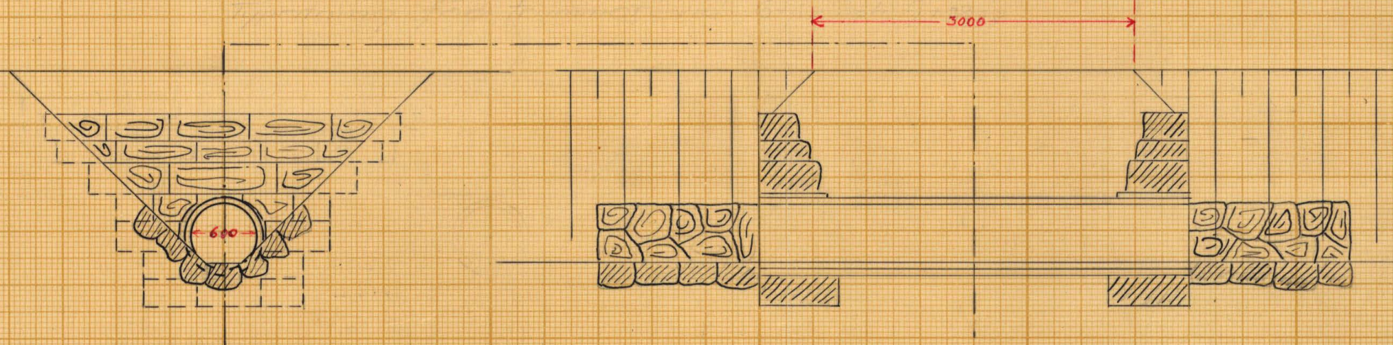
Typritning för trummor vid 6+62 och 9+12
