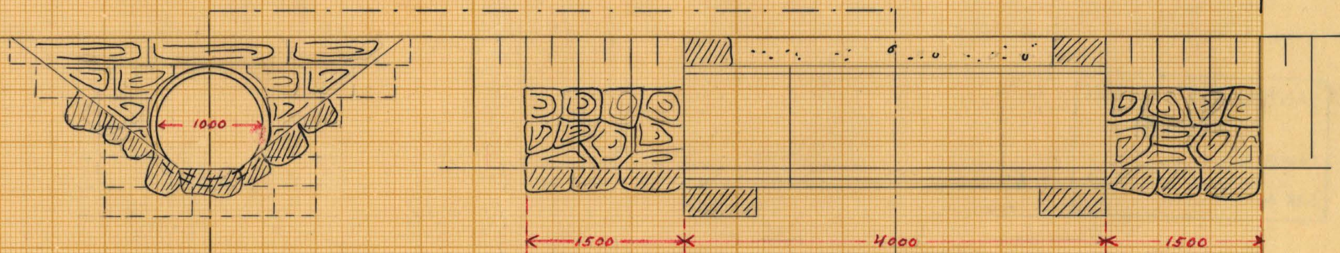
Förslag till trumma vid 0+72
