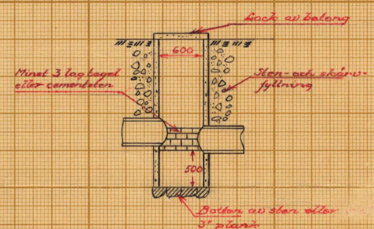
Förslag till brunn med intag vid C.
