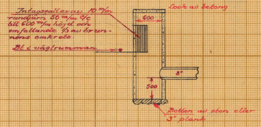
Förslag till brunn med intag vid C.
