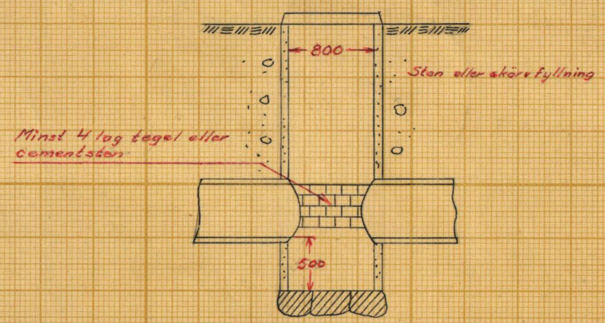
Typritning för brunnar
