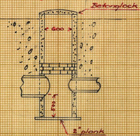
Typritning för brunnar
