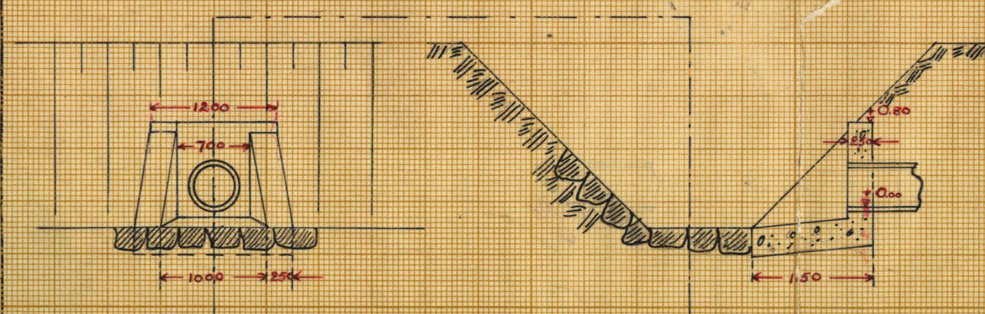
Typritning för rörutlopp.
