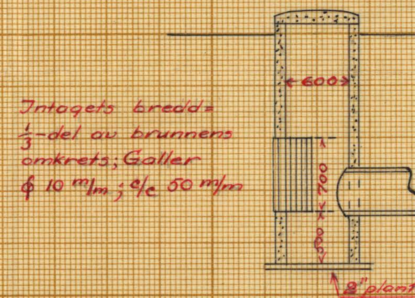
Förslag till brunn med intag
