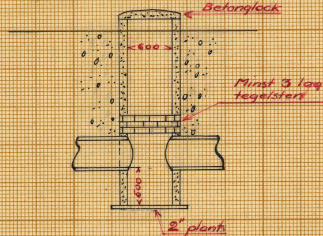
Typritning för brunnar
