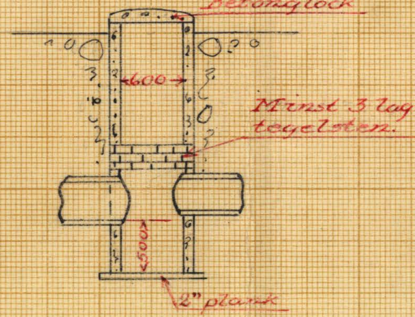
Typritning för brunnar
