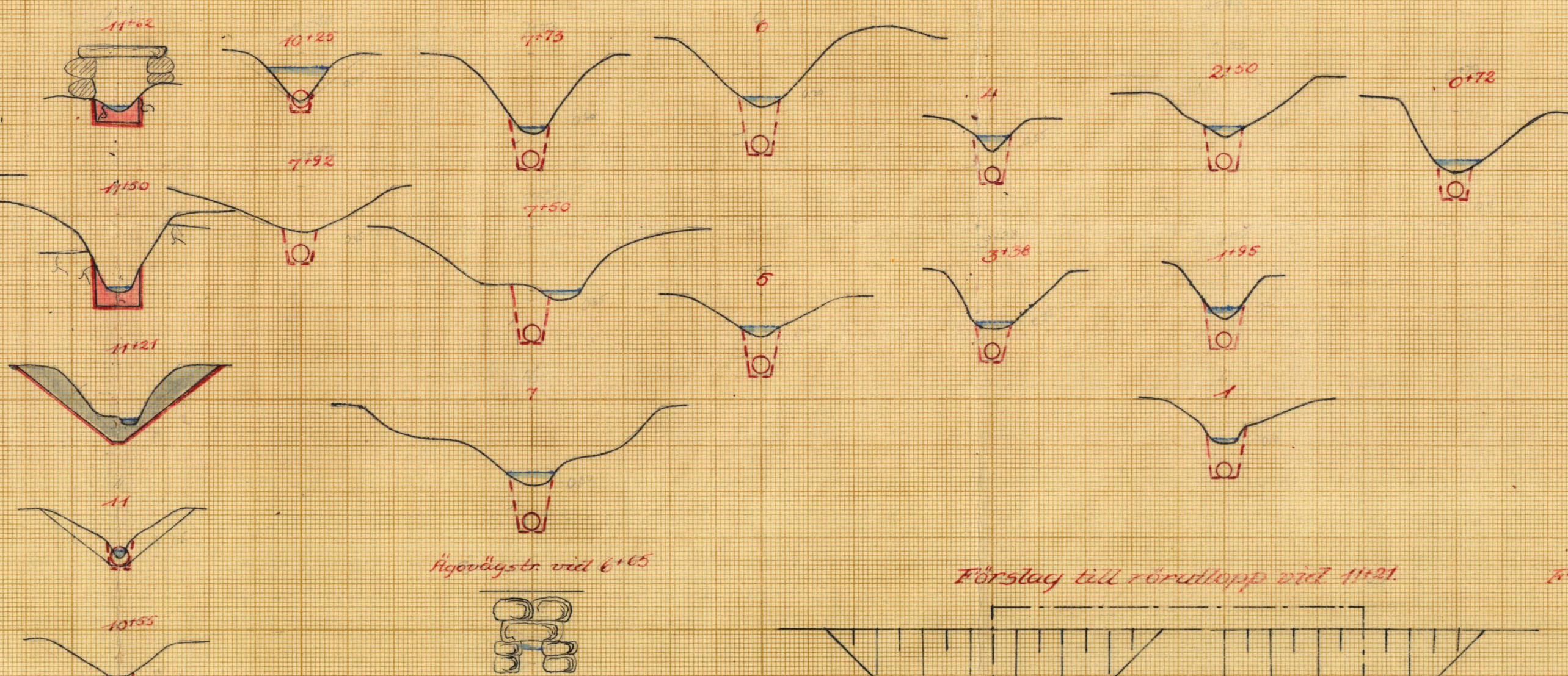
Typritning för brunnar
