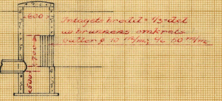
Förslag till kopplingsbrunn vid 4+00
