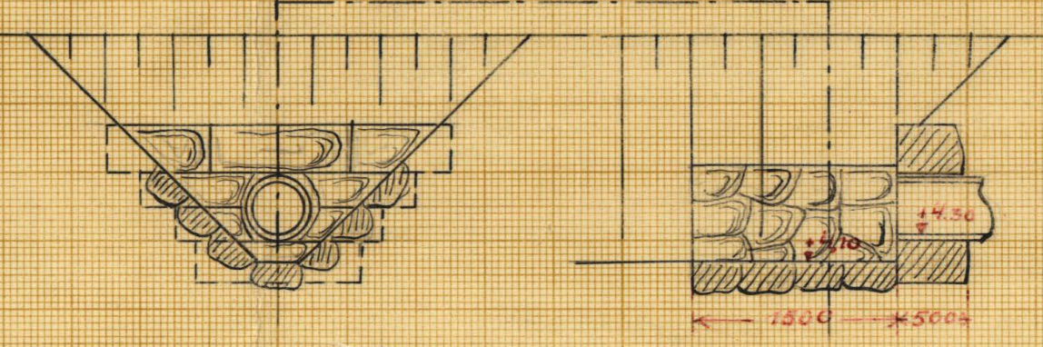
Förslag till rörelsebro vid 11+21
