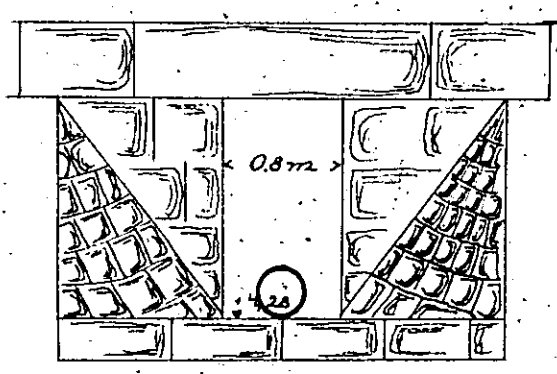
Befintlig landsvägstrumma vid 8+7-25.
