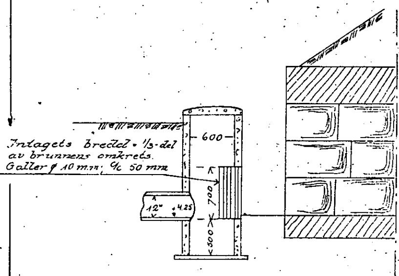
Befintlig landsvägstrumma, bibehålles i oförändrat skick.
