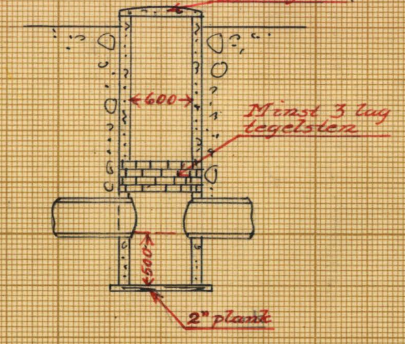
Förslag till brunnar
