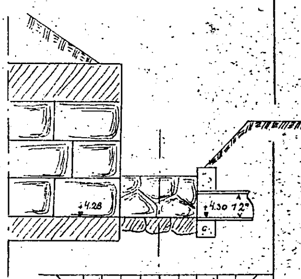
Befintlig landsvägstrumma, bibehålles i oförändrat skick.
