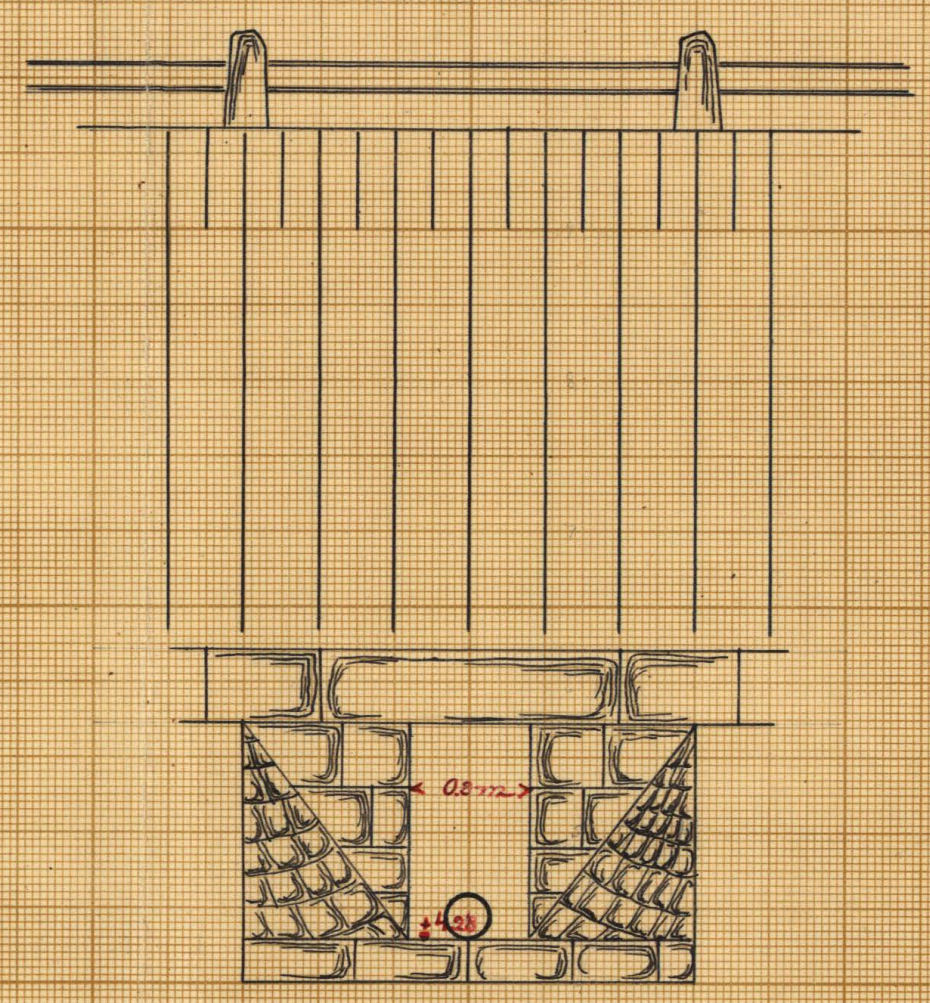
Befintlig landsvägstrumma vid 8+7.25
