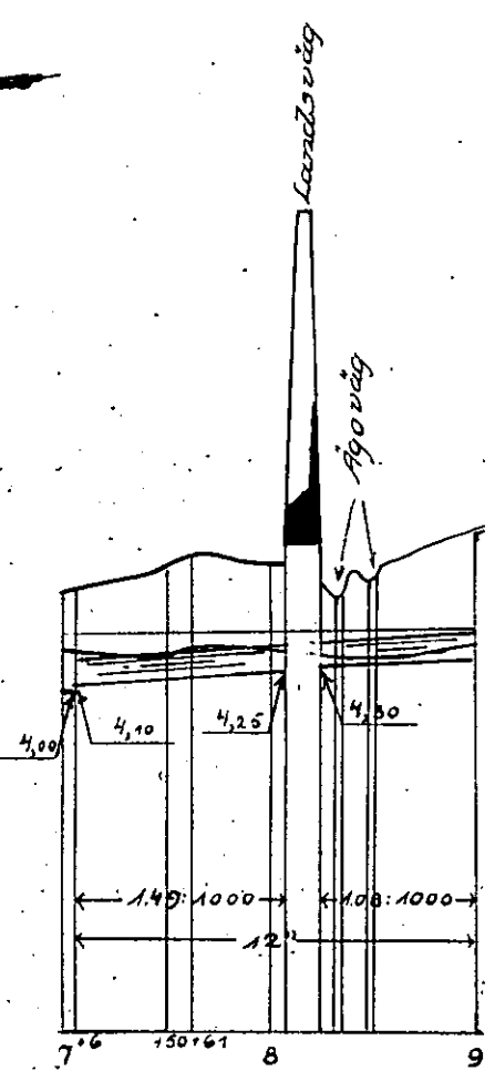
Befintlig landsvägstrumma vid 8+7-25.
