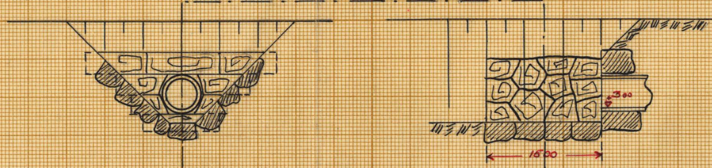
Förelag till rörutlopp vid 0+50
