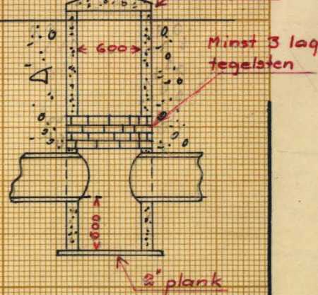
Typpritning för brunnar
