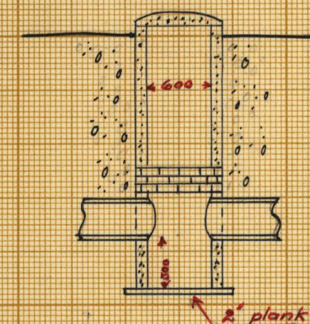
Typritning för brunnar.
