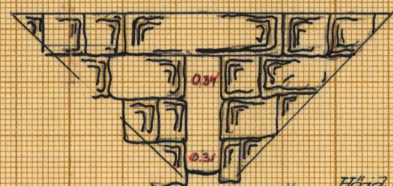
Nedströms trumöppning, vid 1+19. Skala 1:50
