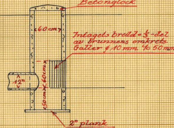
Typritning för brunnar med inlag Belonglock
