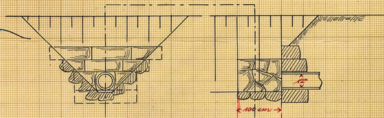
Typritning för rörutlopp.
