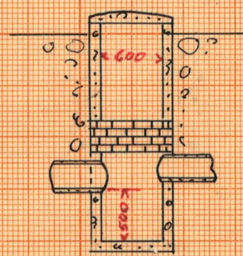
Typritning för brunnar
