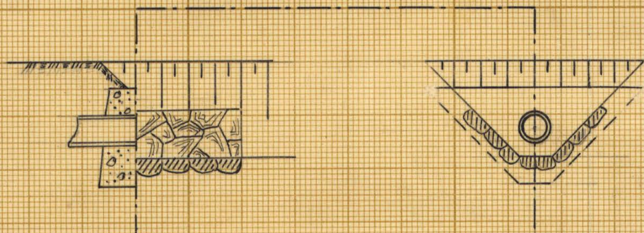
Förslag till rörutlopp vid 0'00
