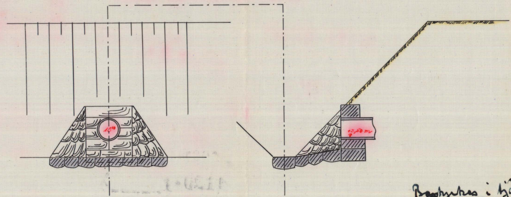
Förslag till rörutlopp vid A.
