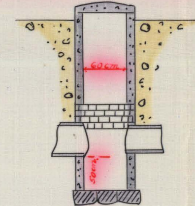
Typritning för brunnar
