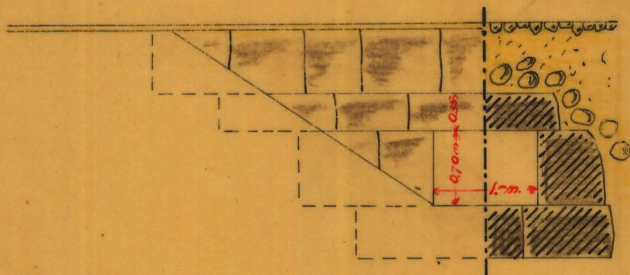
Trummo vid 4+30.
