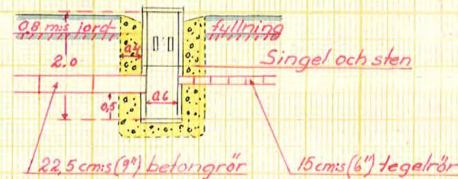
Sektion F och G
