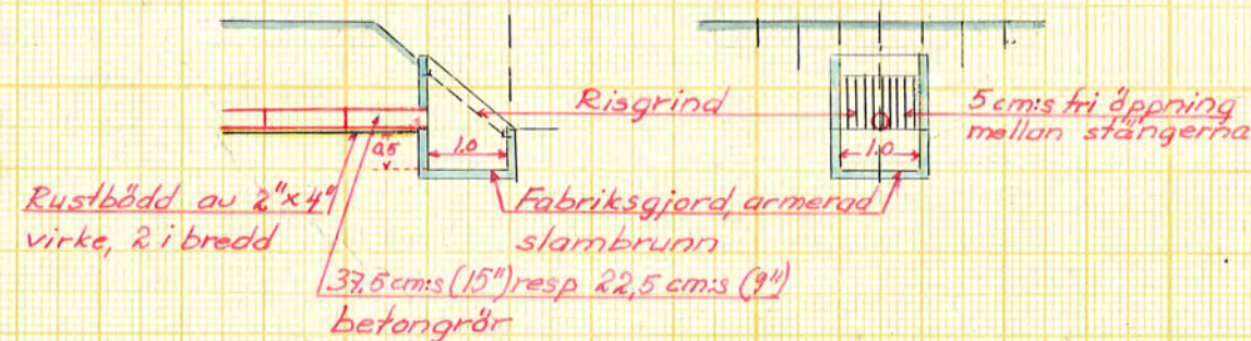
Sektion C' och E'
