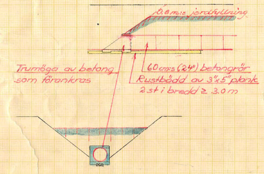
Sektion B
