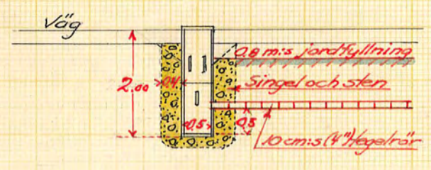
Sektion F.
