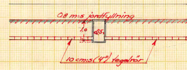
Sektion 11+54
