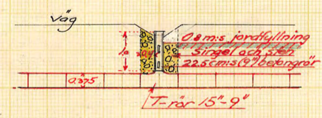
Sektion 5+28
