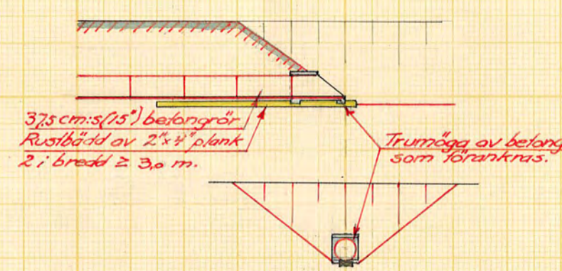
Sektion C.
