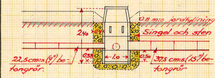
Sektion C.
