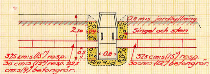
Sektion 4+76,5+35,15+90 5 G.
