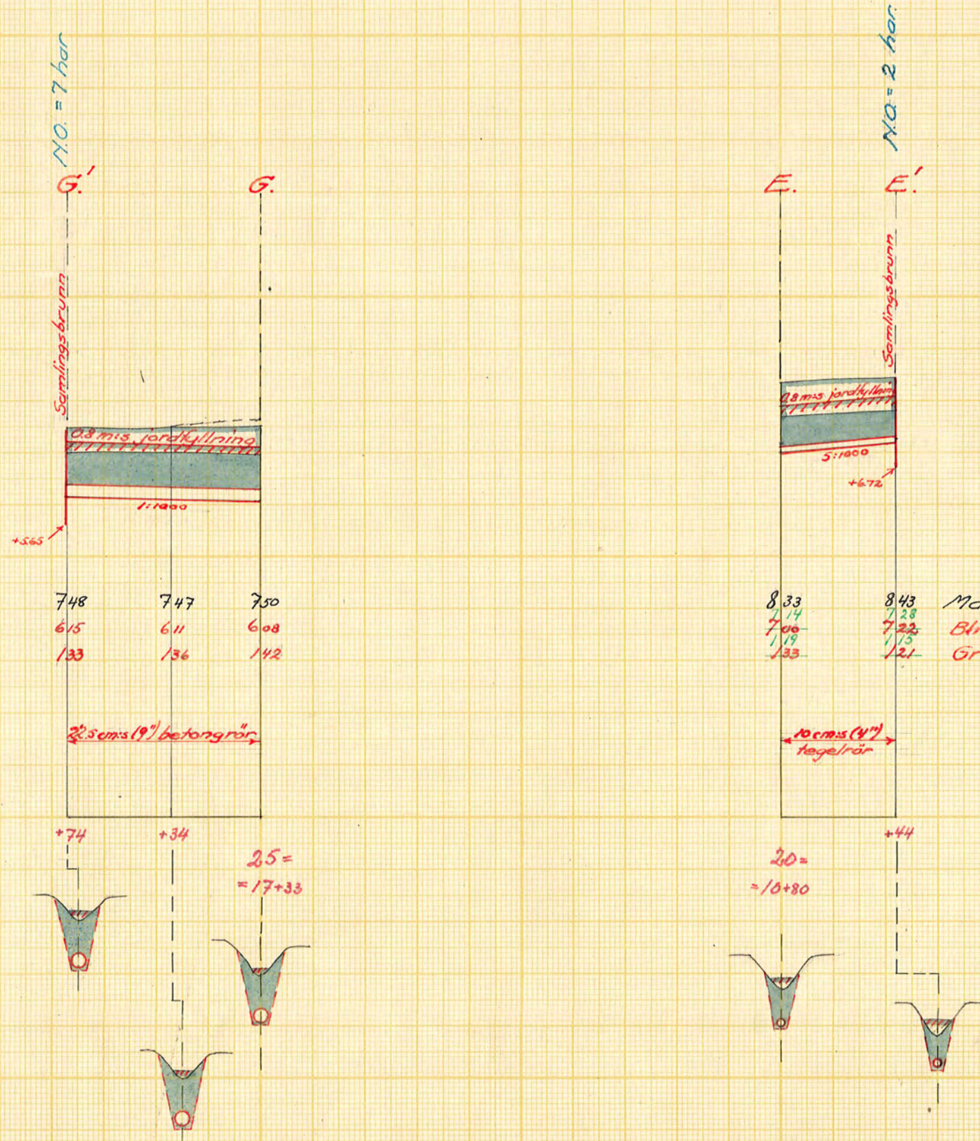
Sektion E.
