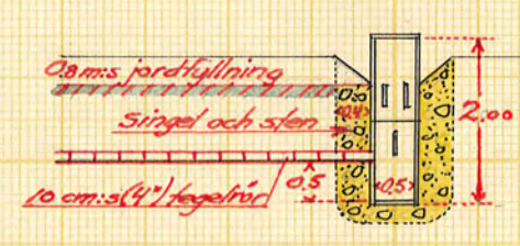
Sektion E.
