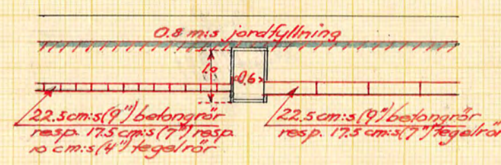
Sektion 7+46,9+52 5 E
