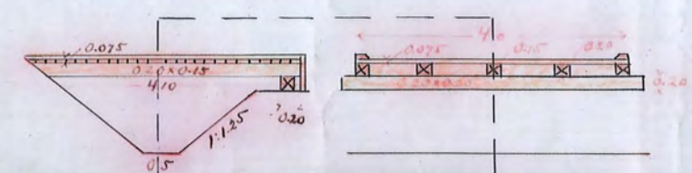
Ägarevägsbroar vid 180 +49 och 124 +54
