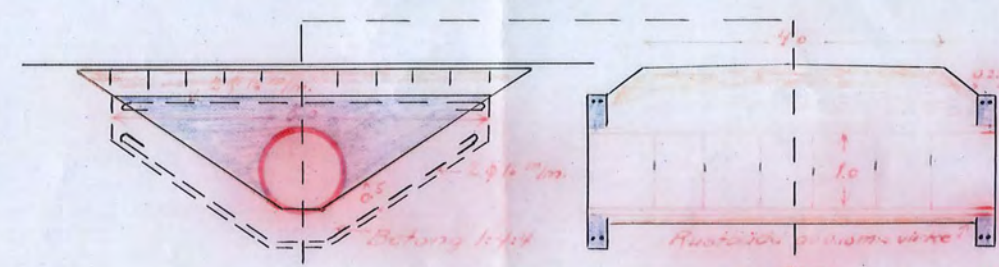
Trumma för utfartsväg vid 85 +16
