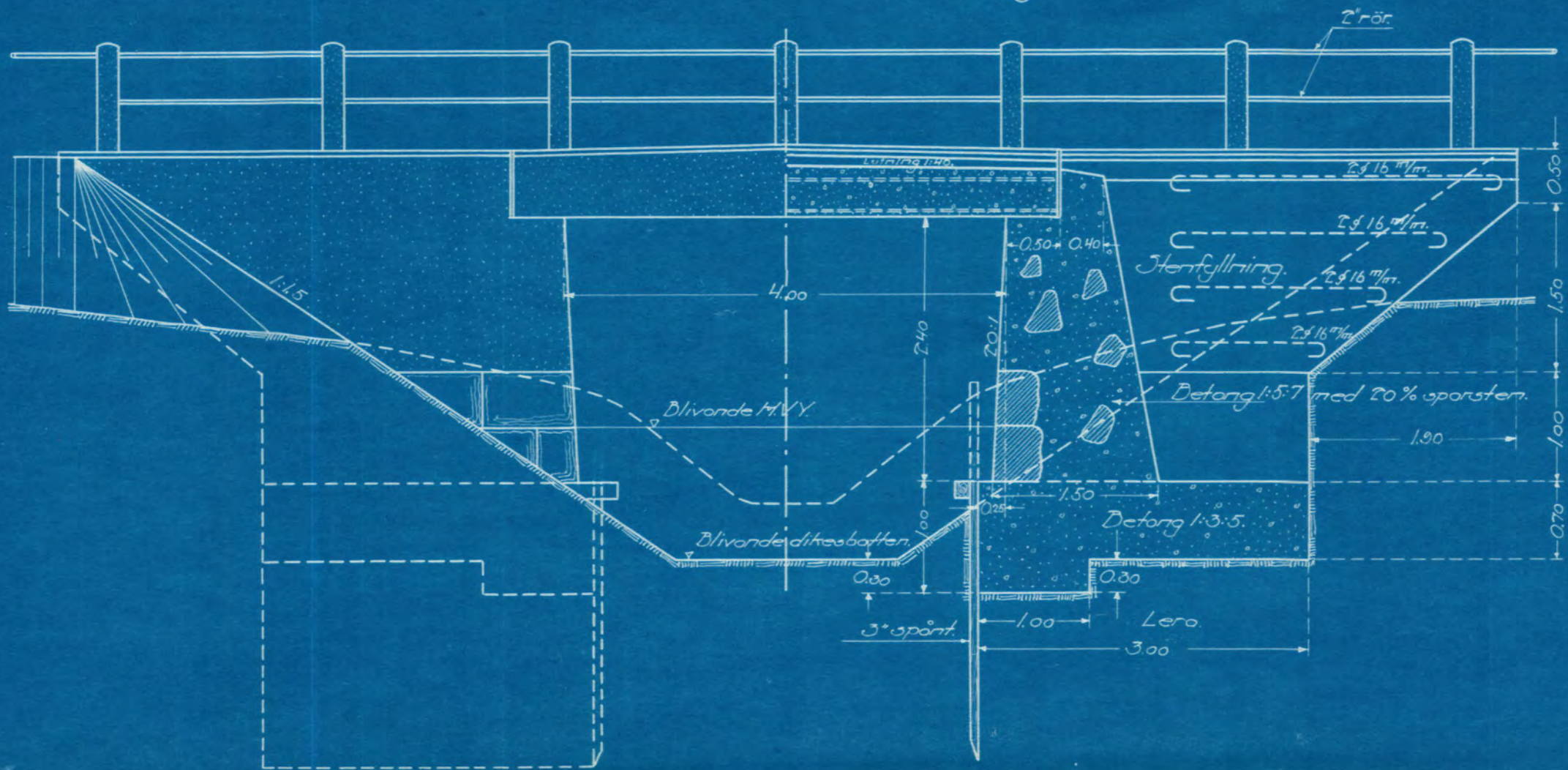
Längdsektion.
