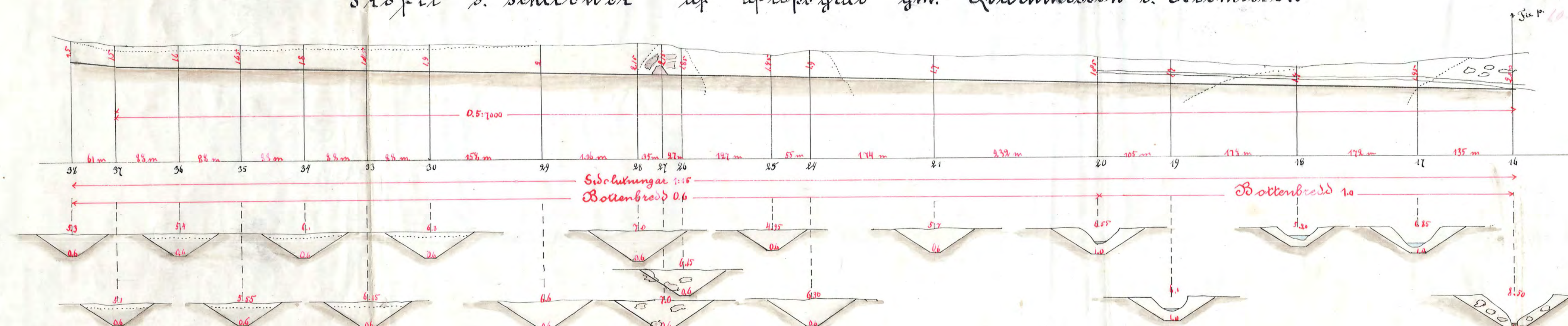
Profil o. skttoner af aflopsgrav gm. Quarmossen o. Rødmosse
