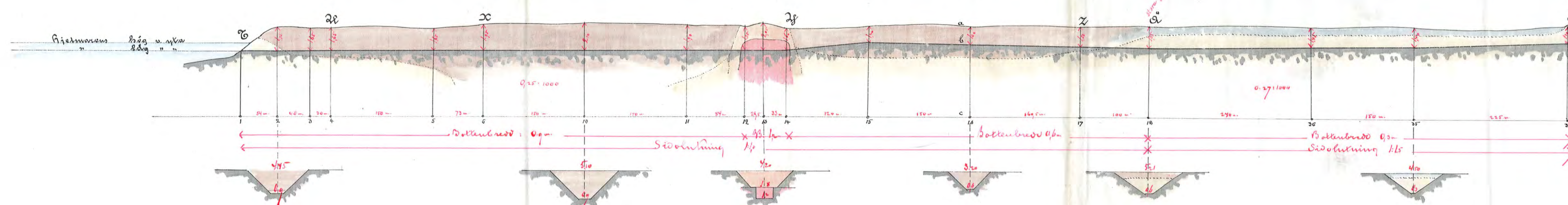
Профил och sektionen af aflopsgraven G-H-X-Y-Z-A-Ä genom Holmstråken
