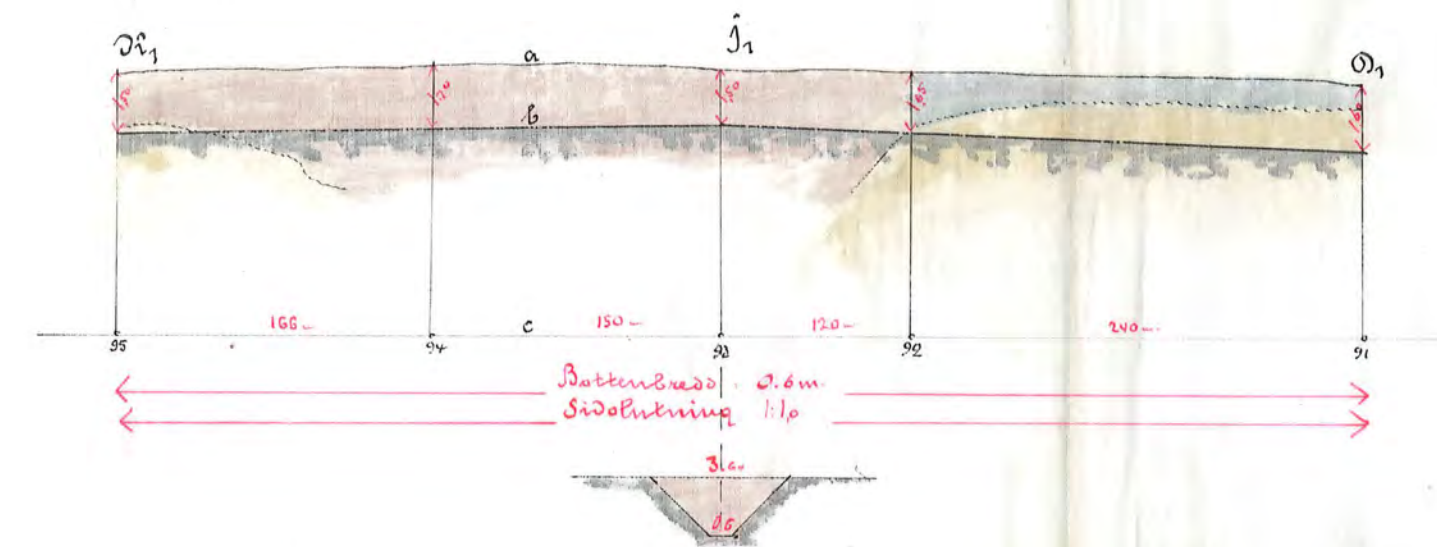
Profil och sektion af aflopsgrav. D 1 -I 1 -O 1
